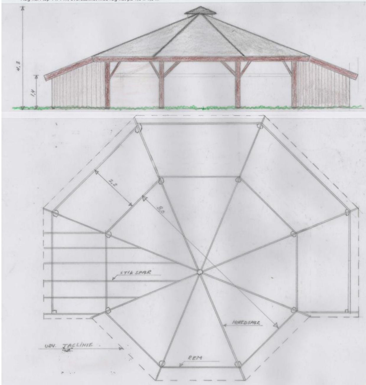
Tegning og beskrivelse af bålhytte med fem tilbygninger fra Shelterbyg.dk.
